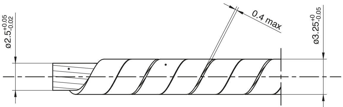
Cavo armato \varnothing 3.25 doppio avvolgimento Double wrapped armoured cable \varnothing 3.25
