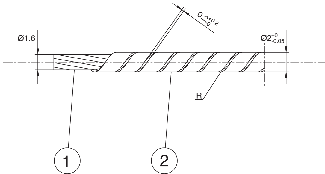
Rope Ø 1.6 - Fune Ø 1.6
